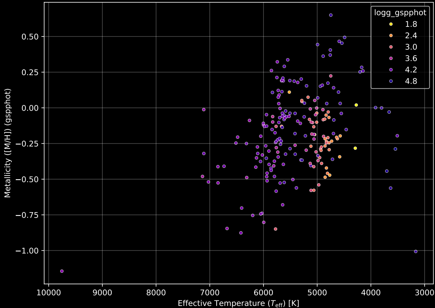
APOGEE DR17 Field: [265-37-O_TESS] Stellar Population Parameters (n= 205)
